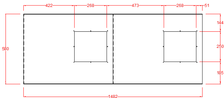
Vista interna base
