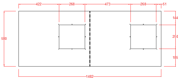
Vista interna base
