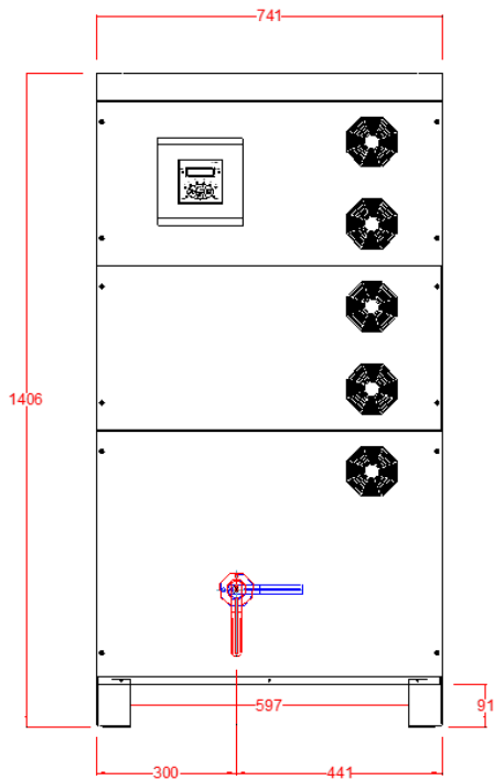
Vista frontale
