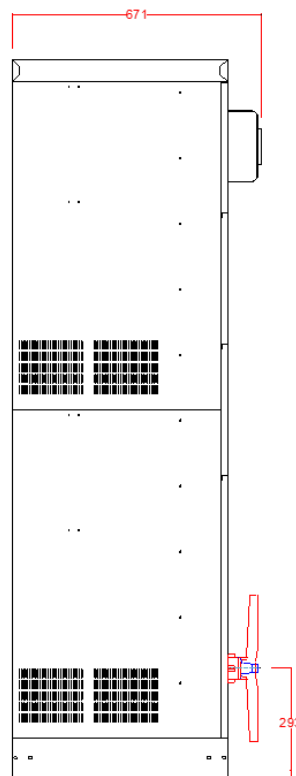
Vista laterale
