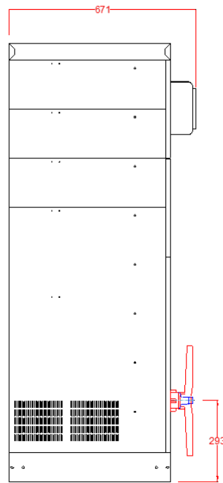
Vista laterale
