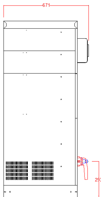
Vista laterale
