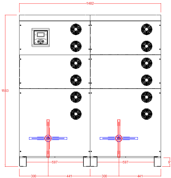
Vista frontale
