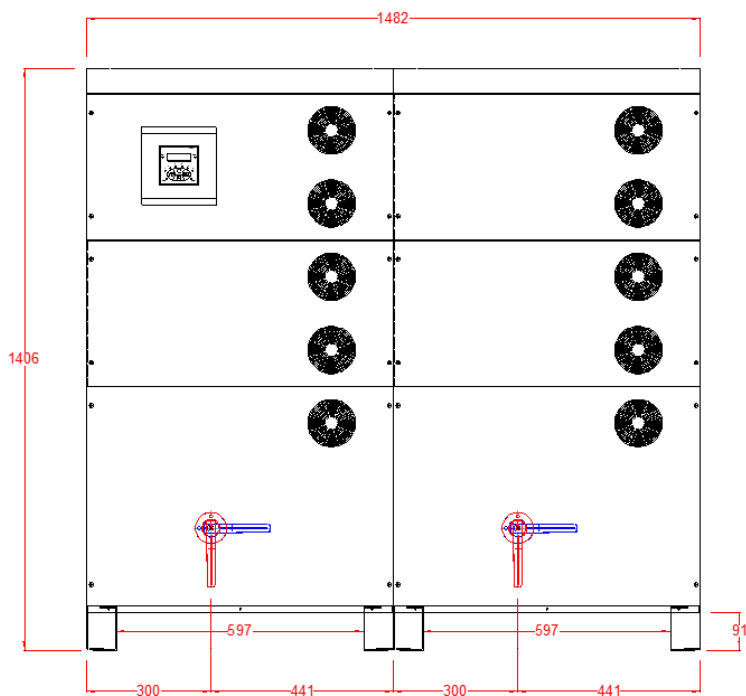
Vista frontale
