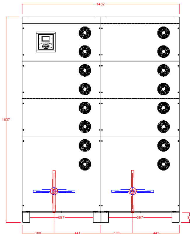
Vista frontale
