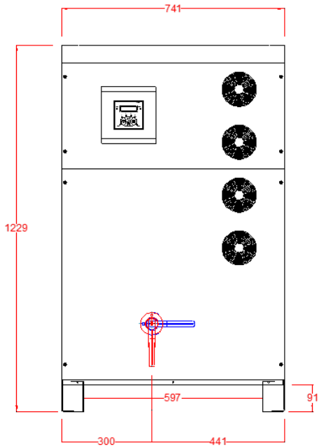
Vista frontale
