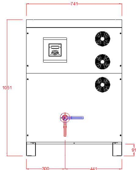
Vista frontale
