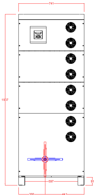
Vista frontale
