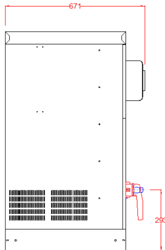
Vista laterale
