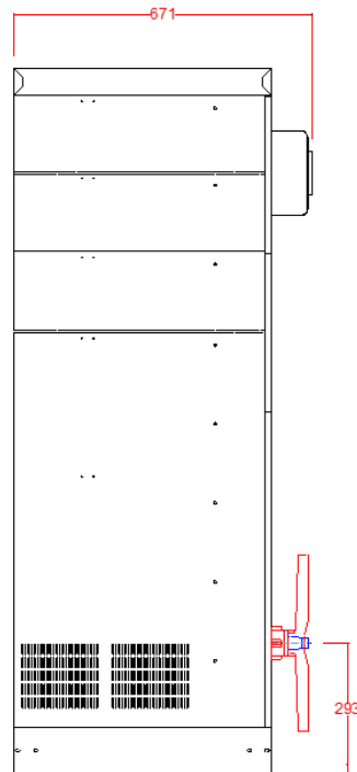
Vista laterale
