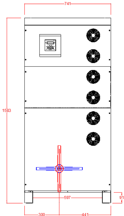
Vista frontale
