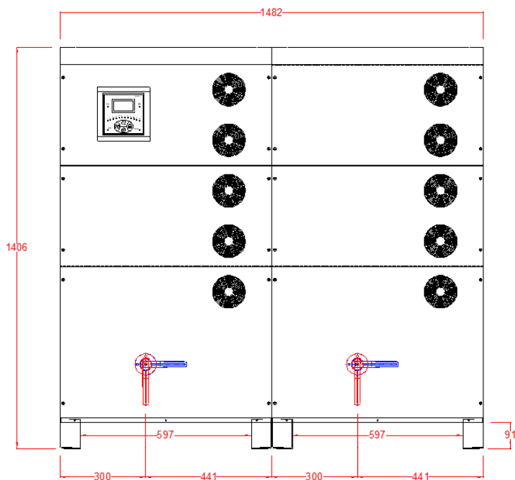
Vista frontale
