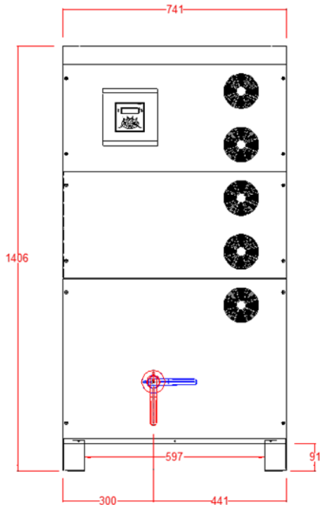
Vista frontale
