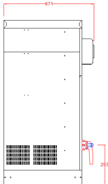
Vista laterale
