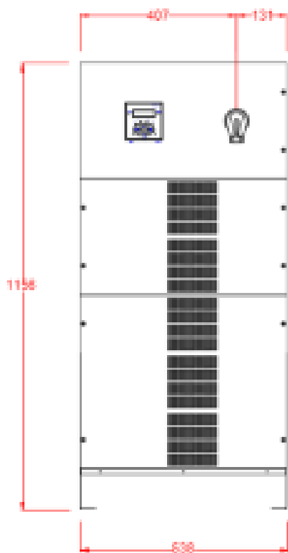
Vista frontale
