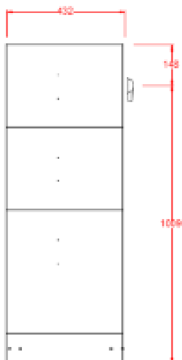
Vista laterale
