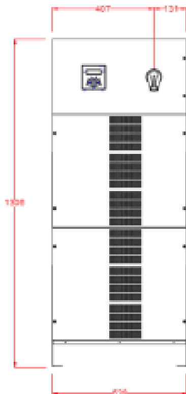
Vista frontale
