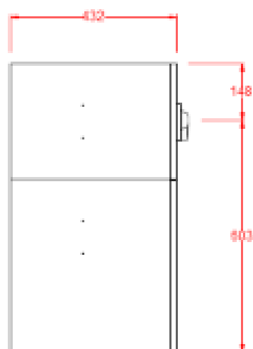
Vista laterale
