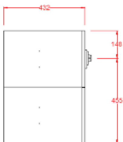
Vista laterale
